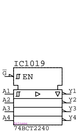
74BCT2240
