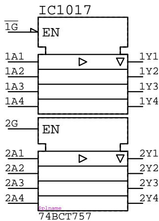
74BCT757
