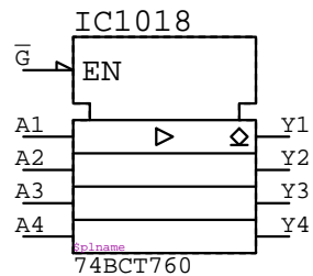
74BCT760
